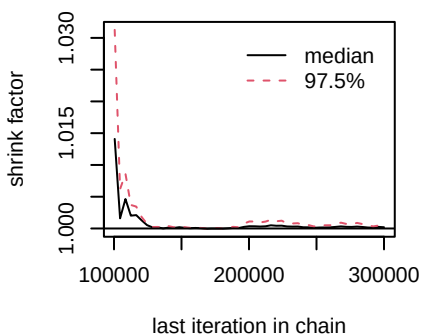
d.Gefitinib.Almonertinib
