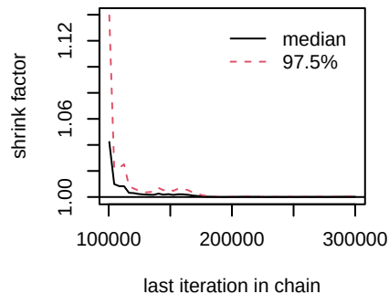
d.Afatinib.Placebo
