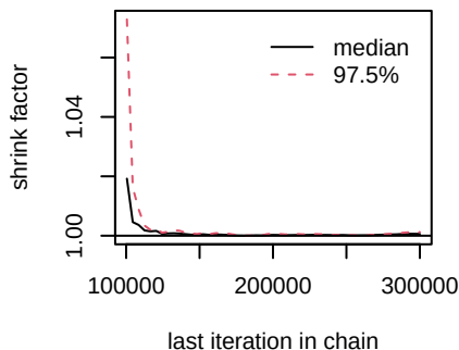
d.Osimertinib.Osimertinib_antiangio
