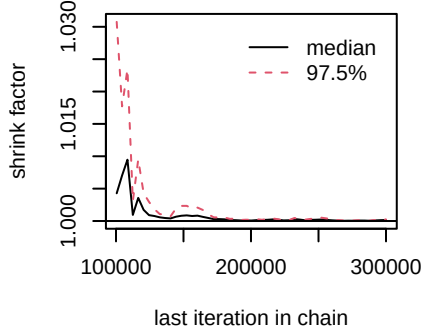
d.Erlotinib.Erlotinib_IGF_1Ri
