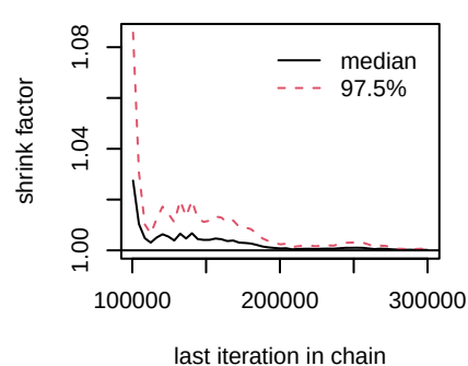
d.Gefitinib.Gefitinib_chemo
