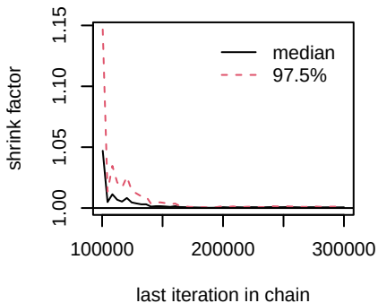
d.Erlotinib.Erlotinib_MMPI
