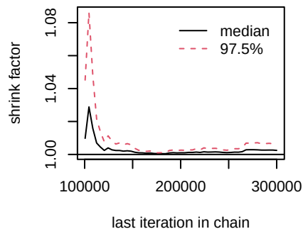
d.chemo.Erlotinib_chemo
