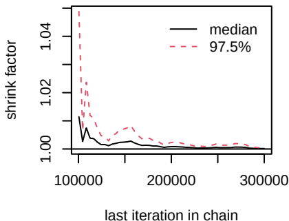
d.Erlotinib.Dacomitinib
