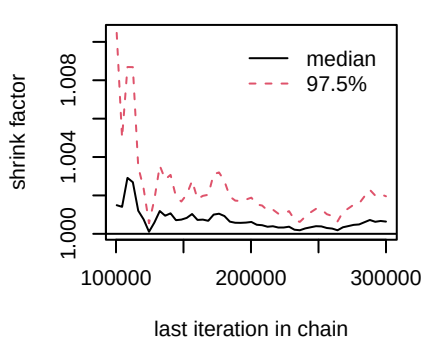
d.Erlotinib.Rociletinib
