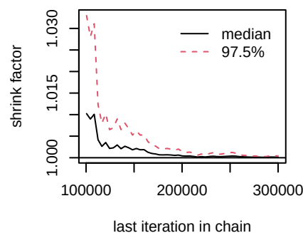
d.Erlotinib.Erlotinib_METi
