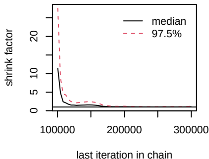
d.Osimertinib.chemo_antiangio
