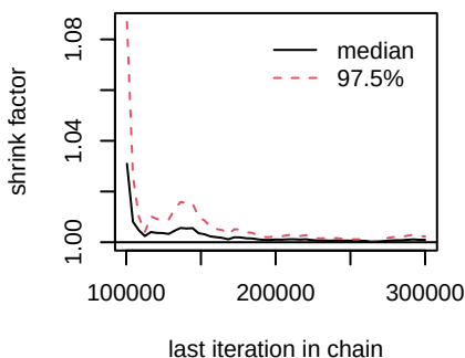
d.Erlotinib.Erlotinib_Autophagy
