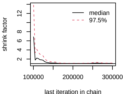
d.Osimertinib.Osimertinib_PD_Ligand
