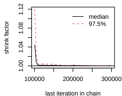
d.Gefitinib_Erlotinib.Zorifertinib
