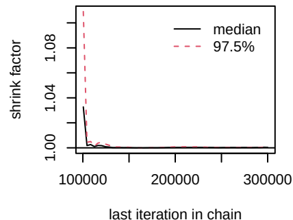
d.Osimertinib.Gefitinib_Erlotinib
