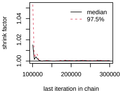
d.Icotinib.Befotertinib
