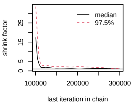
d.Erlotinib.Erlotinib_HGFi
