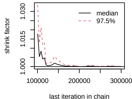
d.Erlotinib.Erlotinib_antiangio
