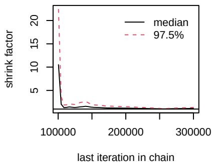
d.Gefitinib.Icotinib
